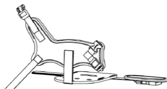
Enkelpositionering inclusief montageplaat
