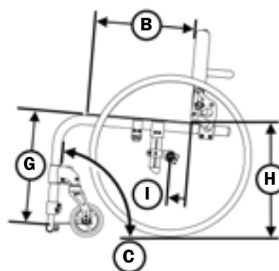
Tekening 3
