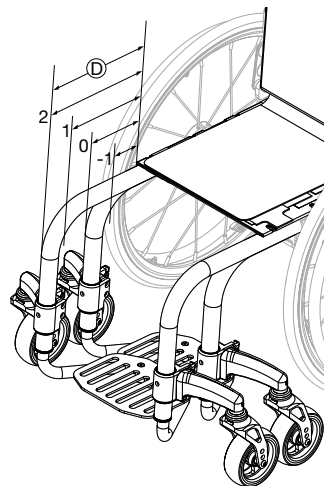
Tekening 3
